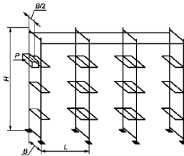
Глубинный стеллаж
