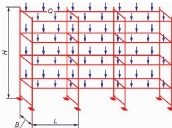
Фронтальный стеллаж
