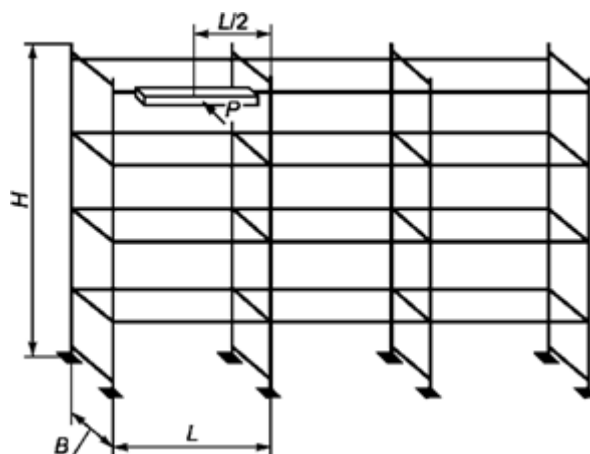
Фронтальный стеллаж
