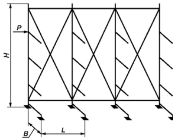
Консольный стеллаж
